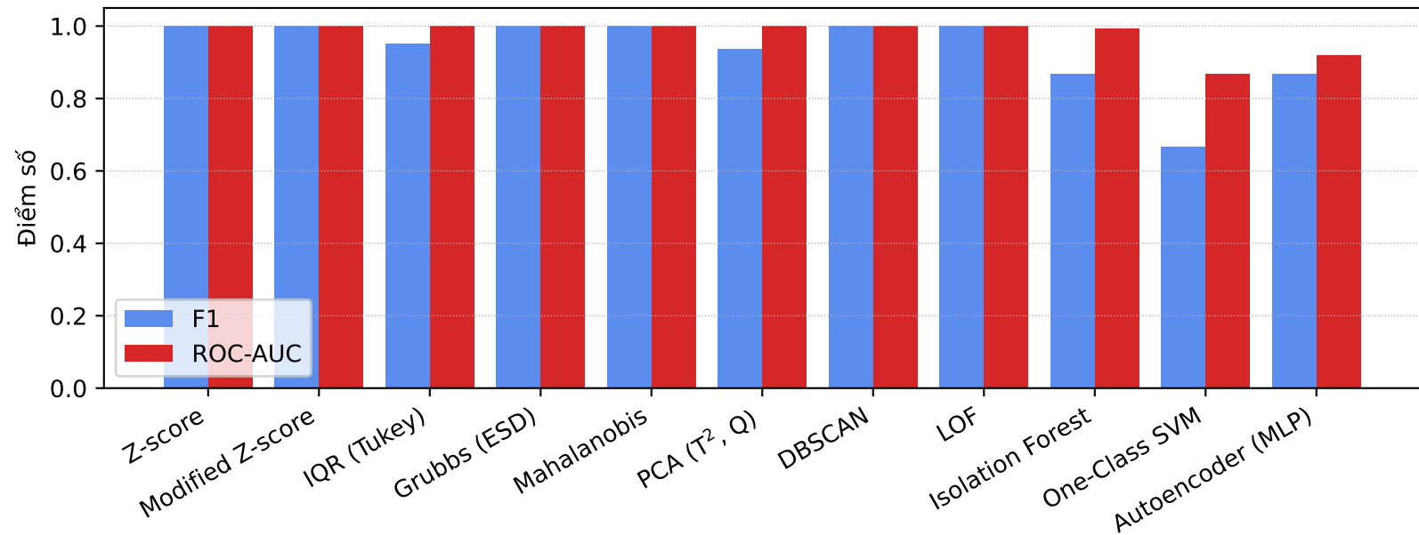
So sánh F1 và ROC-AUC của 11 phương pháp
